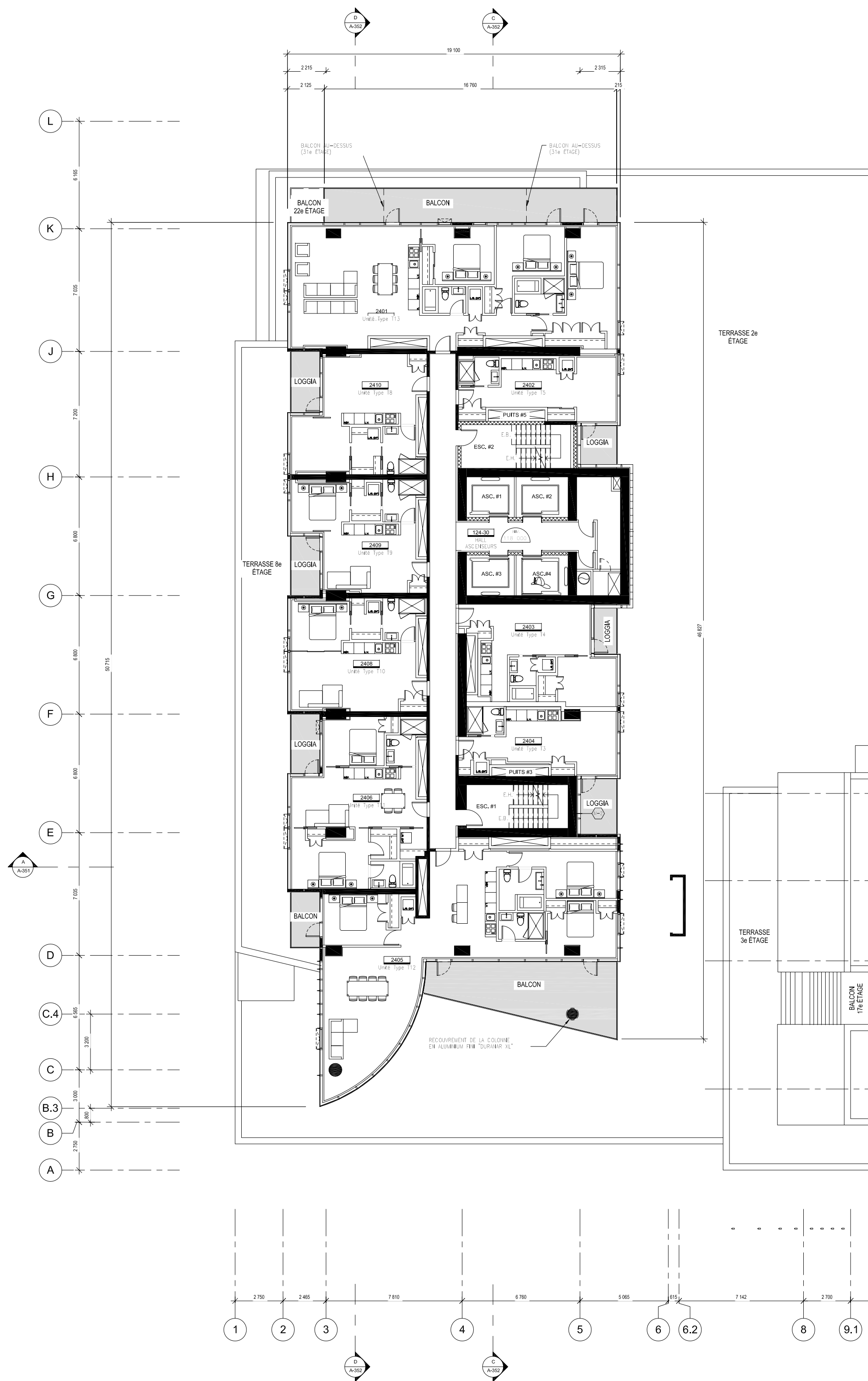
TOUR ICÔNE - 24e ÉTAGE NIVEAU: 110.000mm
